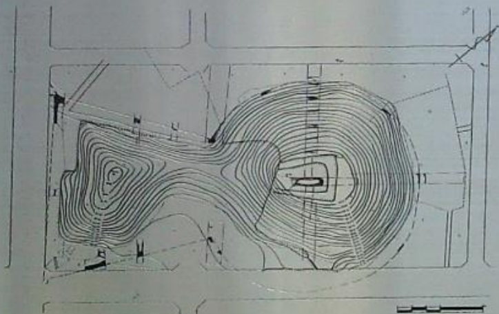
前橋天神山古墳実測測量図
