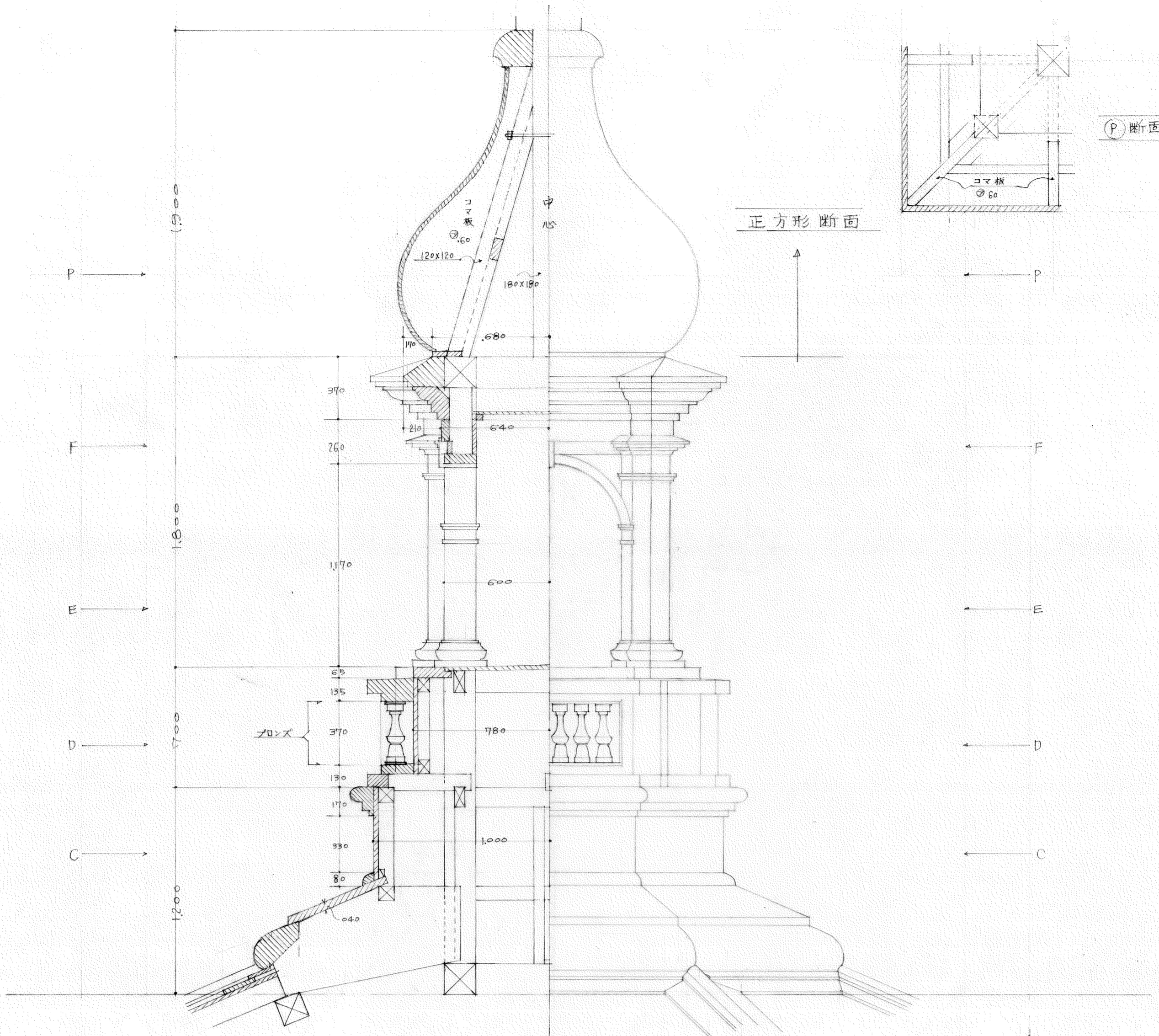
矩計 姿図
