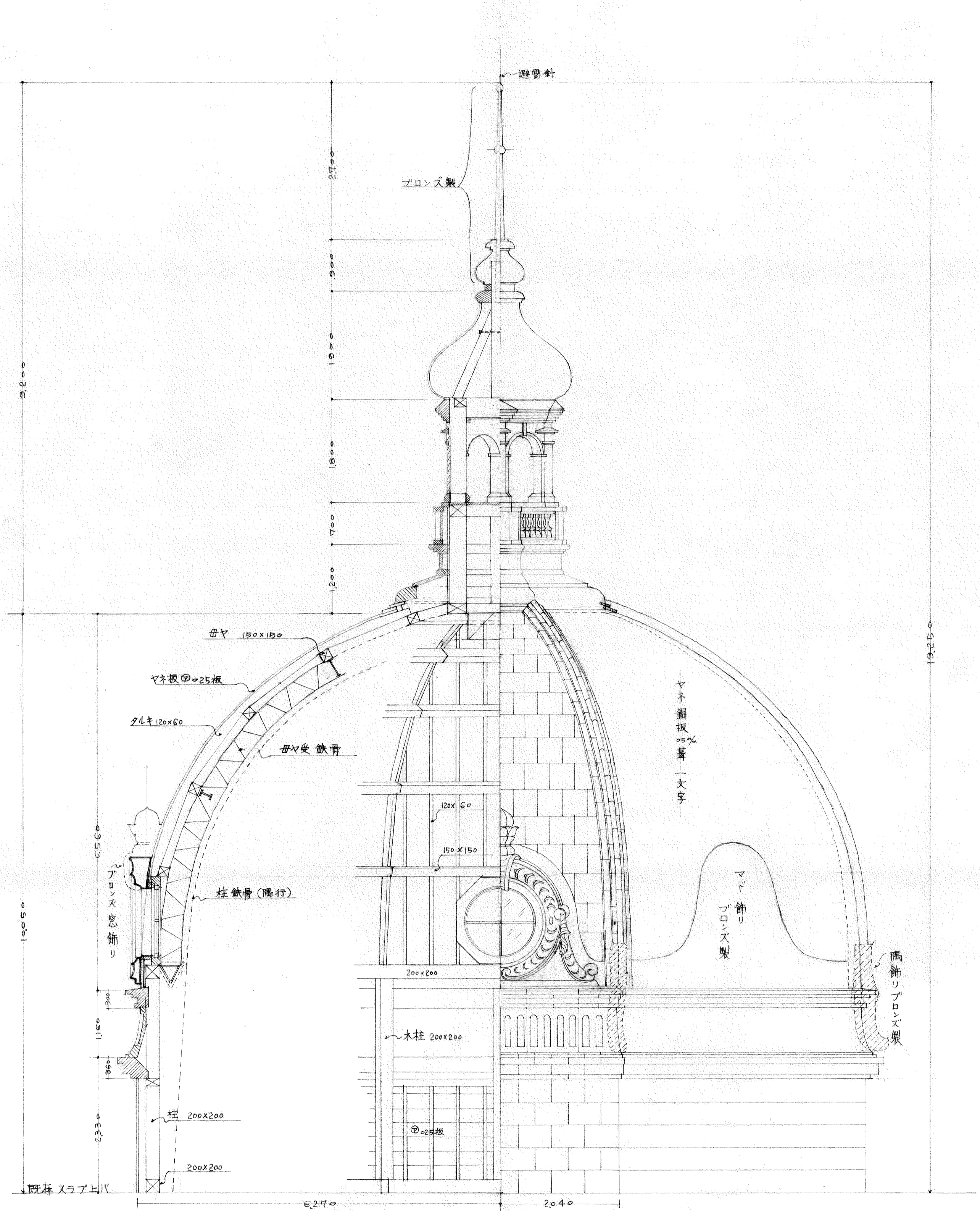
隅切り方向断面
